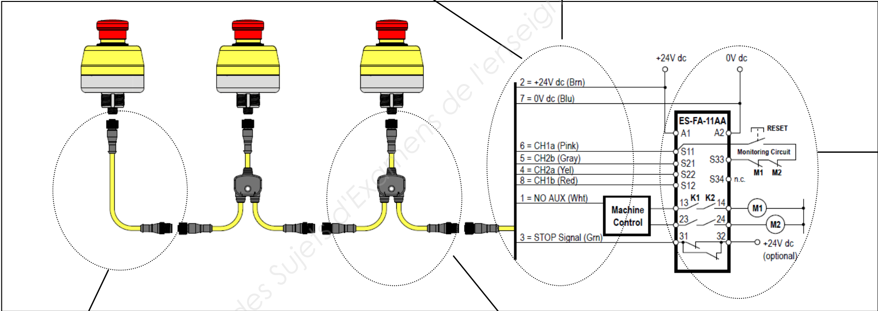
Schéma type de raccordement
